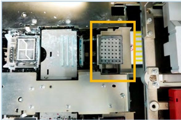
Posizione della spugna di scarico (lato bianco).
